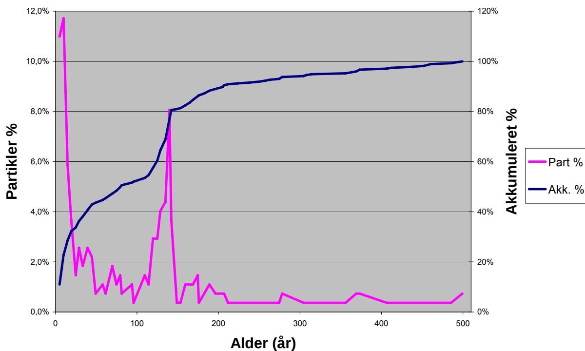
Figur 5.5 Grundvandets aldersfordeling beregnet ud fra partikelbaneberegninger.
